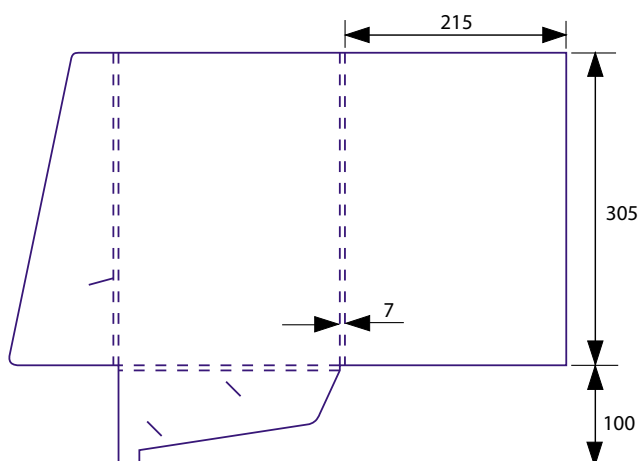
Папка П5. А4, один карман. Клапан замковый. Формат в развернутом виде 545*405 мм.
