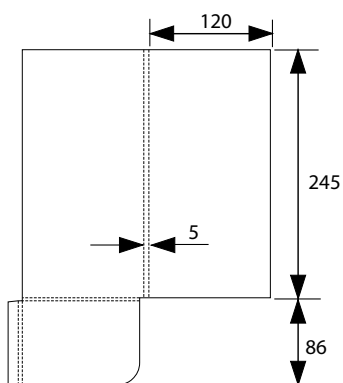
Папка П23. 245x120, один карман. Клапан склейка. Формат в развернутом виде 331*259 мм.
