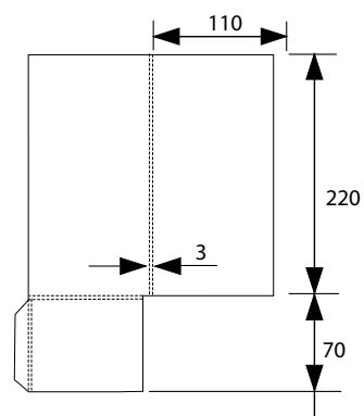
Папка П24. 220x110, один карман. Клапан склейка. Формат в развернутом виде 306*235 мм.
