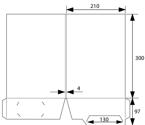
Папка П3. А4, два кармана. Клапана склейка. Диск. Формат в развернутом виде 456*397 мм.
