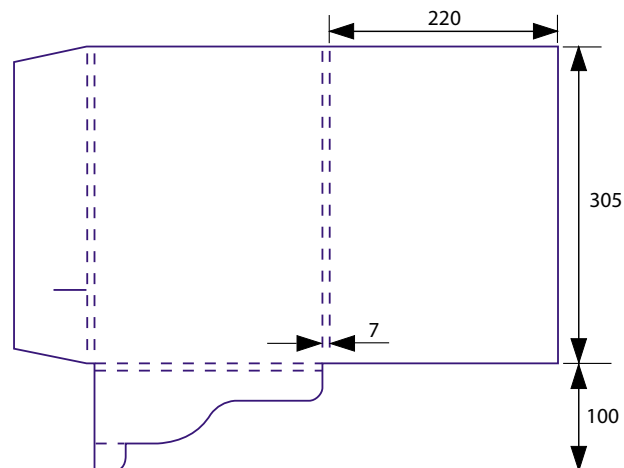
Папка П8. А4, один карман. Клапан замковый. Формат в развернутом виде 525*410 мм.
