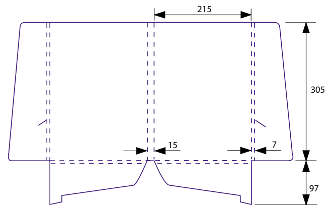
Папка П2. А4, два кармана. Клапаны замковые. Формат в развернутом виде 630*400 мм.
